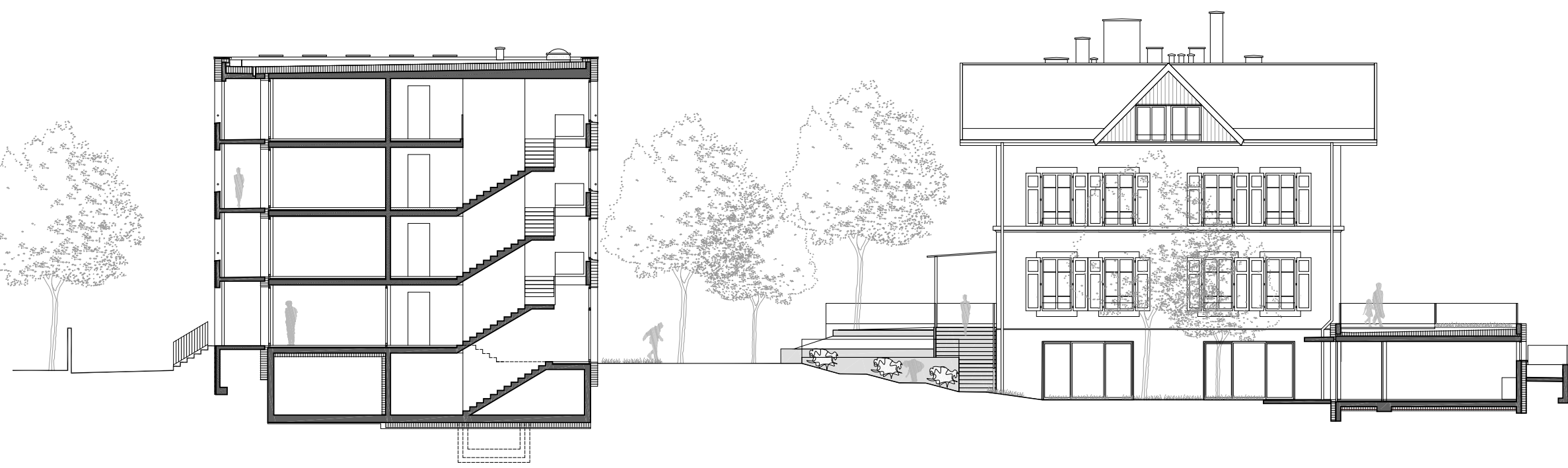
Coupe transversale
